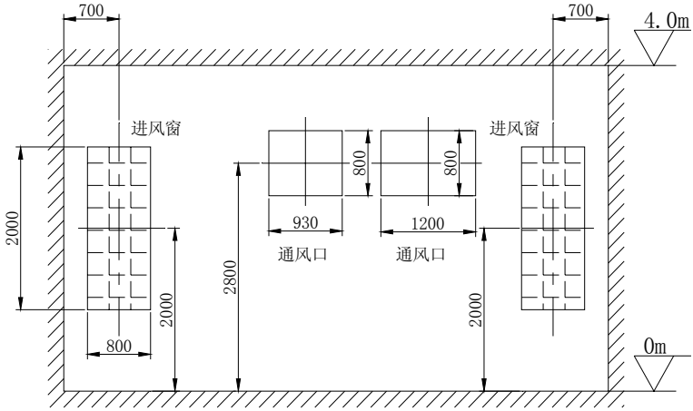
土建布置图(立面视图)
