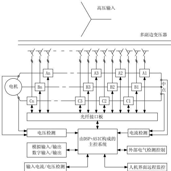
单元串联变频器原理电路
