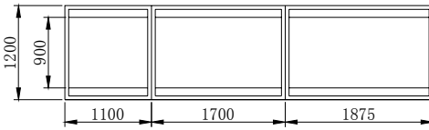
电缆沟道及槽钢基础图
