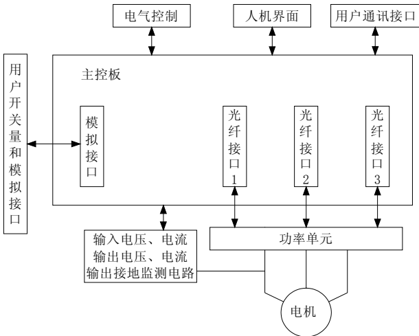
主控系统框图
