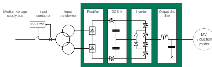
ACS 1000典型框图
