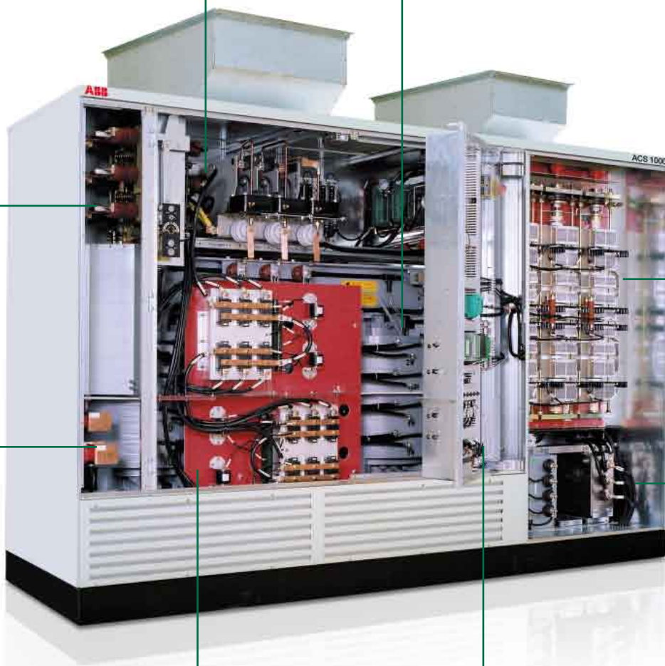
标配的24脉波输入桥
