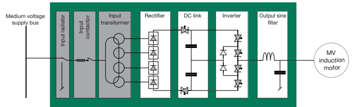
ACS 1000i典型框图
