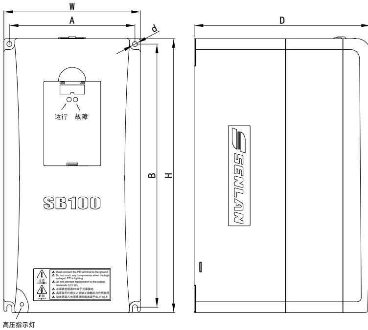
SB100系列变频器的外形尺寸及重量如下表:
