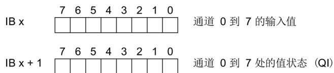
图 4-1 地址空间
