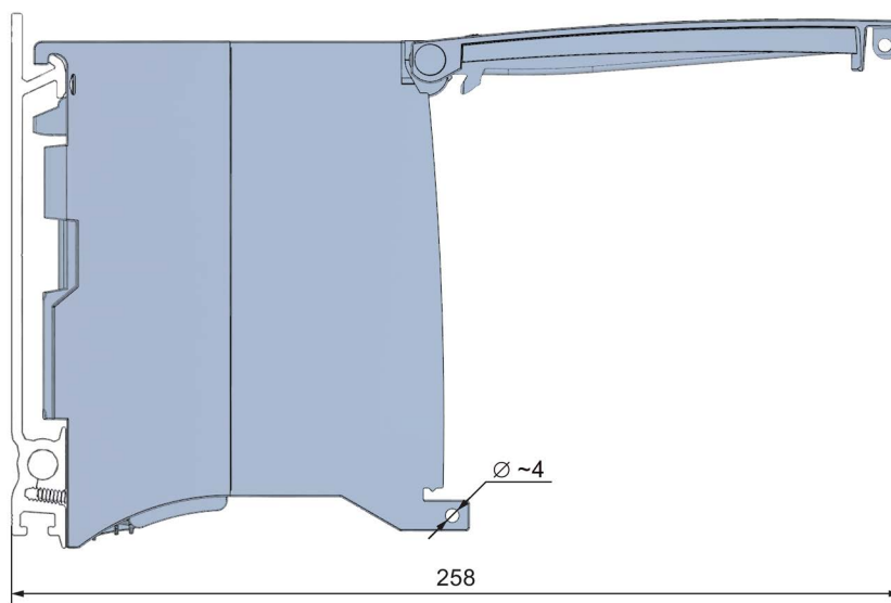
图 A-2 CPU 1511-1 PN 的尺寸图，前面板打开时的侧视图
