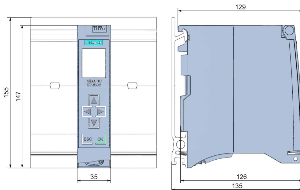
图 A-1 CPU 1511-1 PN 的尺寸图，正视图和侧视图
